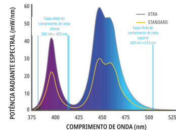
Bandas de comprimentos de onda efetivas para polimerização de compósitos Intervalo de comprimento de onda utilizável: 385 – 515nm
